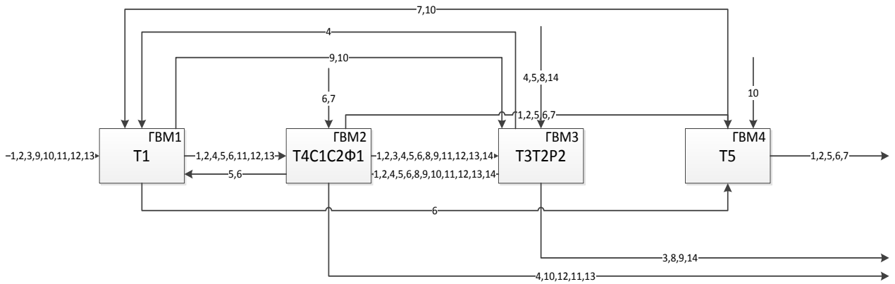
Рис. 1 Організаційно-технологічна схема ГВД
