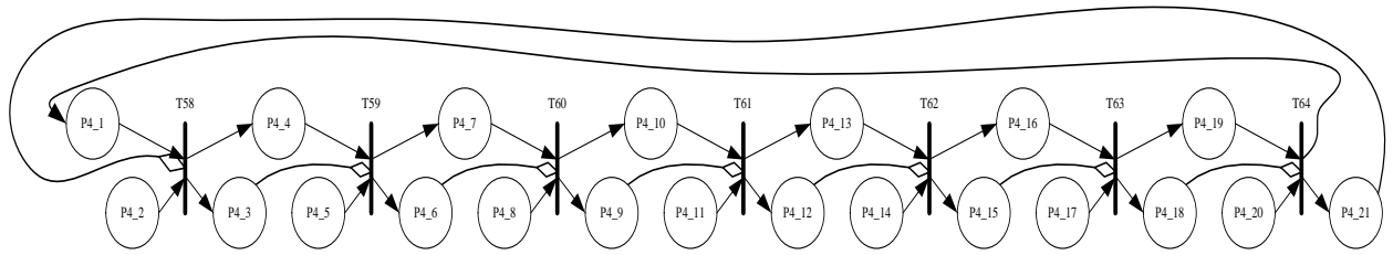
Рис. 11 Модель мережі Петрі для ГВМ4
